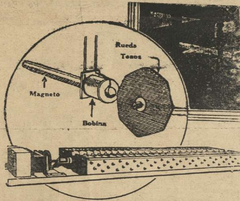
Magneto y rueda de tonos, de las que hay noventa y una, dispuestas en la caja que se ve en la parte inferior del grabado, accionadas todas por un motor, sincrónico.
