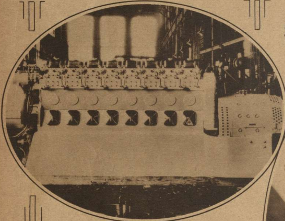
MUEVE UN TREN a dos millas por minuto: Motor Diesel de 600 caballos que suministra la fuerza motriz a un tren hecho totalmente de acero y al cual se ha dado el apropiado nombre de "El Céforo".
