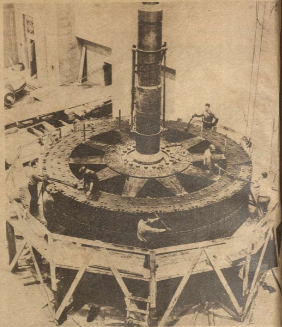
GIGANTESCO GENERADOR ELECTRICO instalado en la Presa Boulder en Estados Unidos, y al que sirve de rotor el enorme aparato que se ve en esta fotografía.
