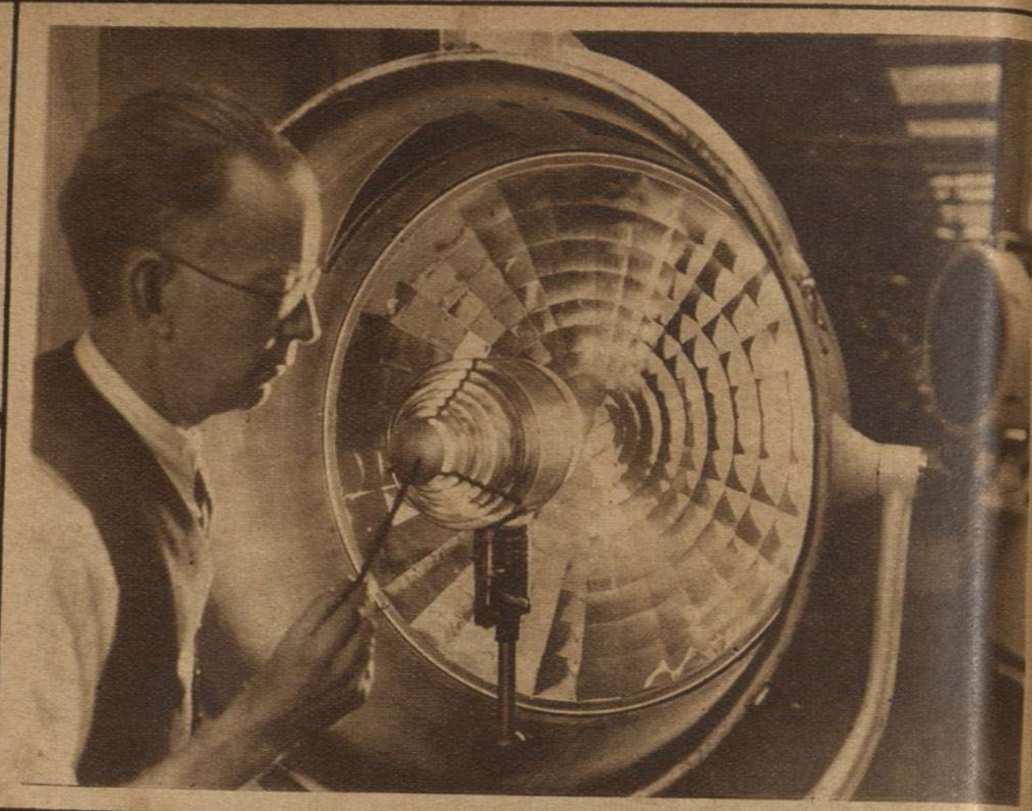
HAROLD FITZGERALD, de Los Angeles, California ha inventado un faro eléctrico que atraviesa las nieblas más espesas a una distancia de 15 kilómetros. Al examinar el aparato se ve que es la fiel reproducción del ojo de una mosca. Los ensayos efectuados han sido completamente satisfactorios.
