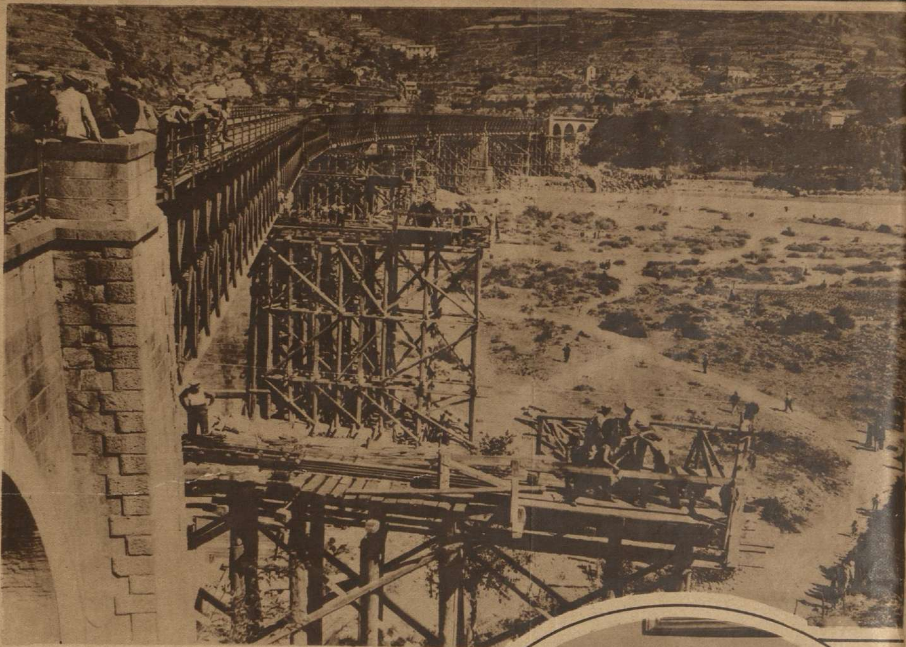
VEINTITRES MINUTOS después de que el último tren había pasado sobre el puente de Borgotaro, Italia, en la línea que va de Parma a Spezzia, se había colocado uno nuevo con peso total de mil setecientas toneladas. Esta fotografía muestra como el nuevo puente de metal, armado sobre los pilares de madera provisionales a la derecha, fué deslizado sobre los arcos de piedra con precisión matemática.
