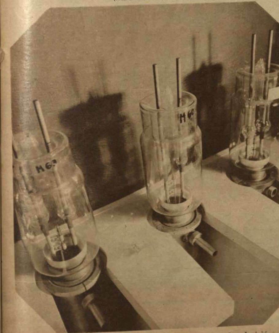
Tubos de alto voltaje empleados en los programas de televisión. (Authenticated News Photo)
