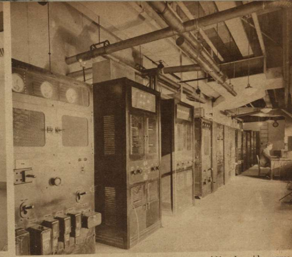
La televisión no sólo trasmite la escena, sino también el sonido correspondiente. He aquí la cámara de control, donde ambas operaciones se refunden en la misma onda eléctrica. (Authenticated News Photo)
