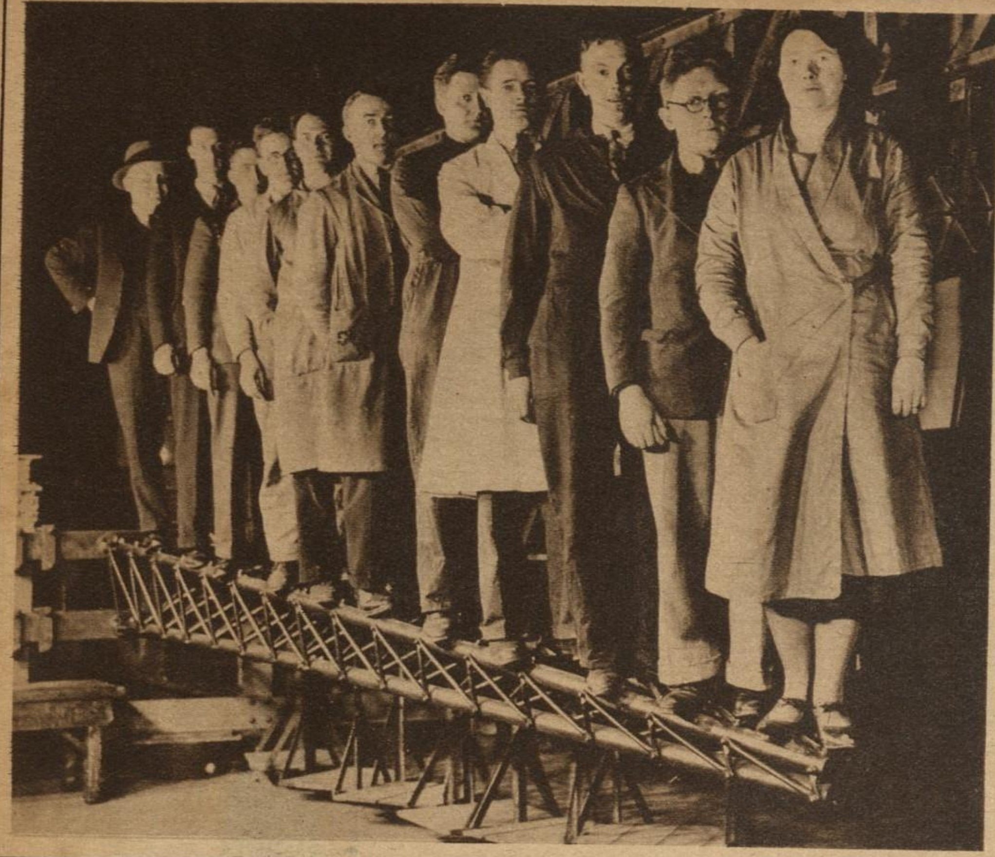
LA ULTIMA PALABRA en técnica aeronáutica consiste en la sustitución de partes de metal fundido, por tuercas y tornillos. Los innovadores de este procedimiento demuestran que la resistencia no disminuye, como parece probarlo este ensayo en que vemos once personas de pie sobre la extremidad de un ala.
