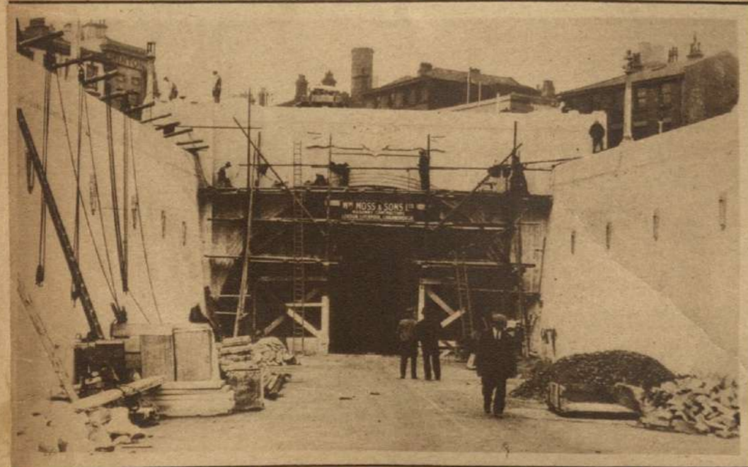
UN GRAN TUNEL CASI TERMINADO: Se trata del Tunnel del Mersey, en Liverpool, Inglaterra y esta fotografía fué tomada en la entrada de Dale Street, de la grandiosa obra de canalización.
