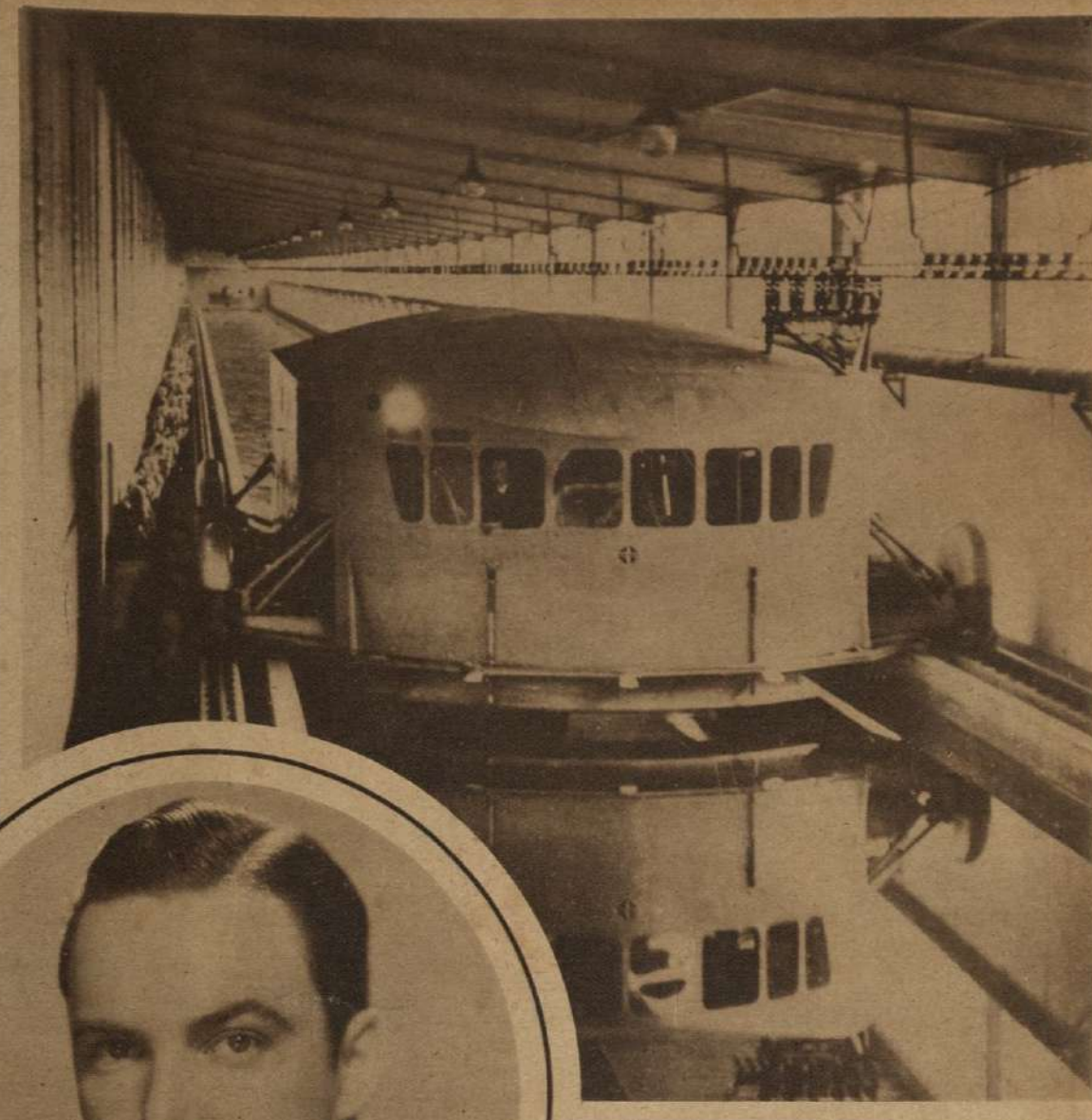
EN EL INSTITUTO EXPERIMENTAL DE HAMBURGO, se ha construido este tunel de 320 metros de largo, destinado a probar la resistencia y capacidad de los hidroaviones. Vemos al centro la locomotora destinada a tirar de los aparatos para estudiar la resistencia del agua.
